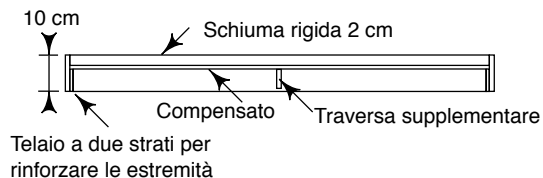
Schema costruttivo alleggerito
